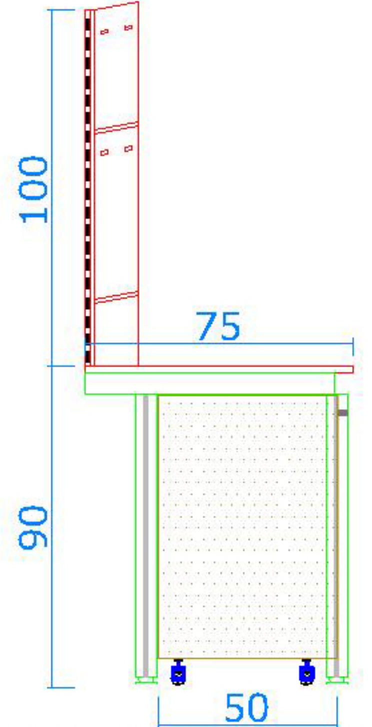
-U- AYAK KENAR TEZGAH YAN GÖRÜNÜŞ VE KESİTLERİ
