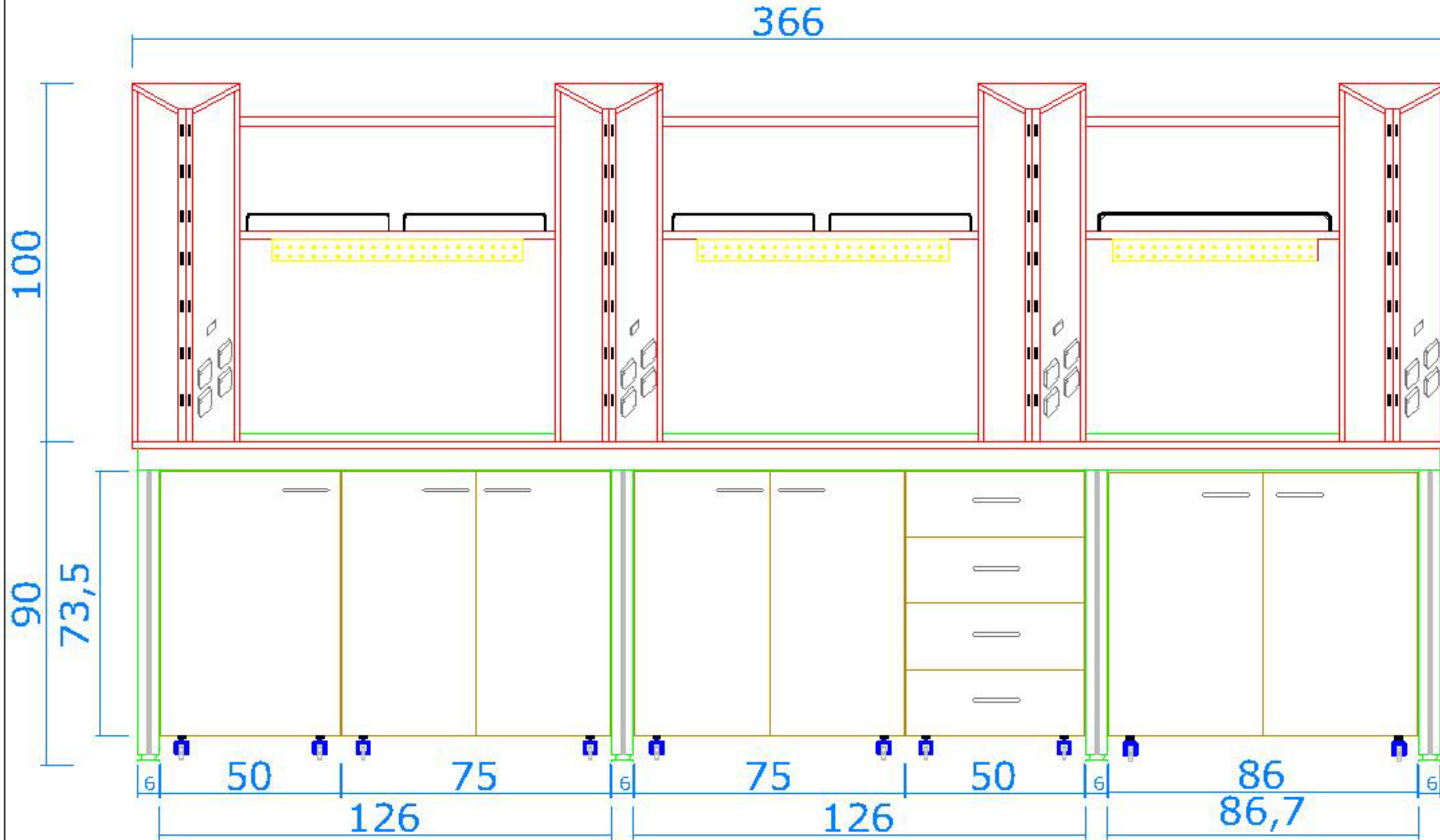
-U- AYAK KENAR TEZGAH ÖN GÖRÜNÜŞ VE KESİTLERİ
